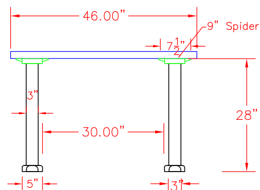
Budget Edge Metal T Bases
