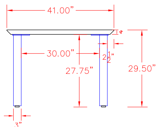
Deluxe Edge Metal Legs
