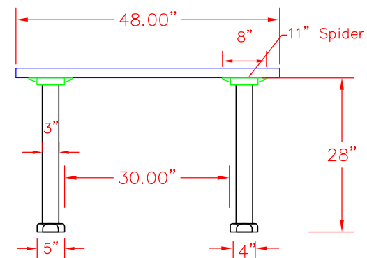
Deluxe Edge Metal T Bases
